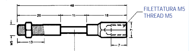
MOLLA DI DISASSAMENTO DISASSAMENTO MAX 3 mm MIS - ALIGNEMENT SPRING MAX MIS. - ALIGNEMENT 3 mm
